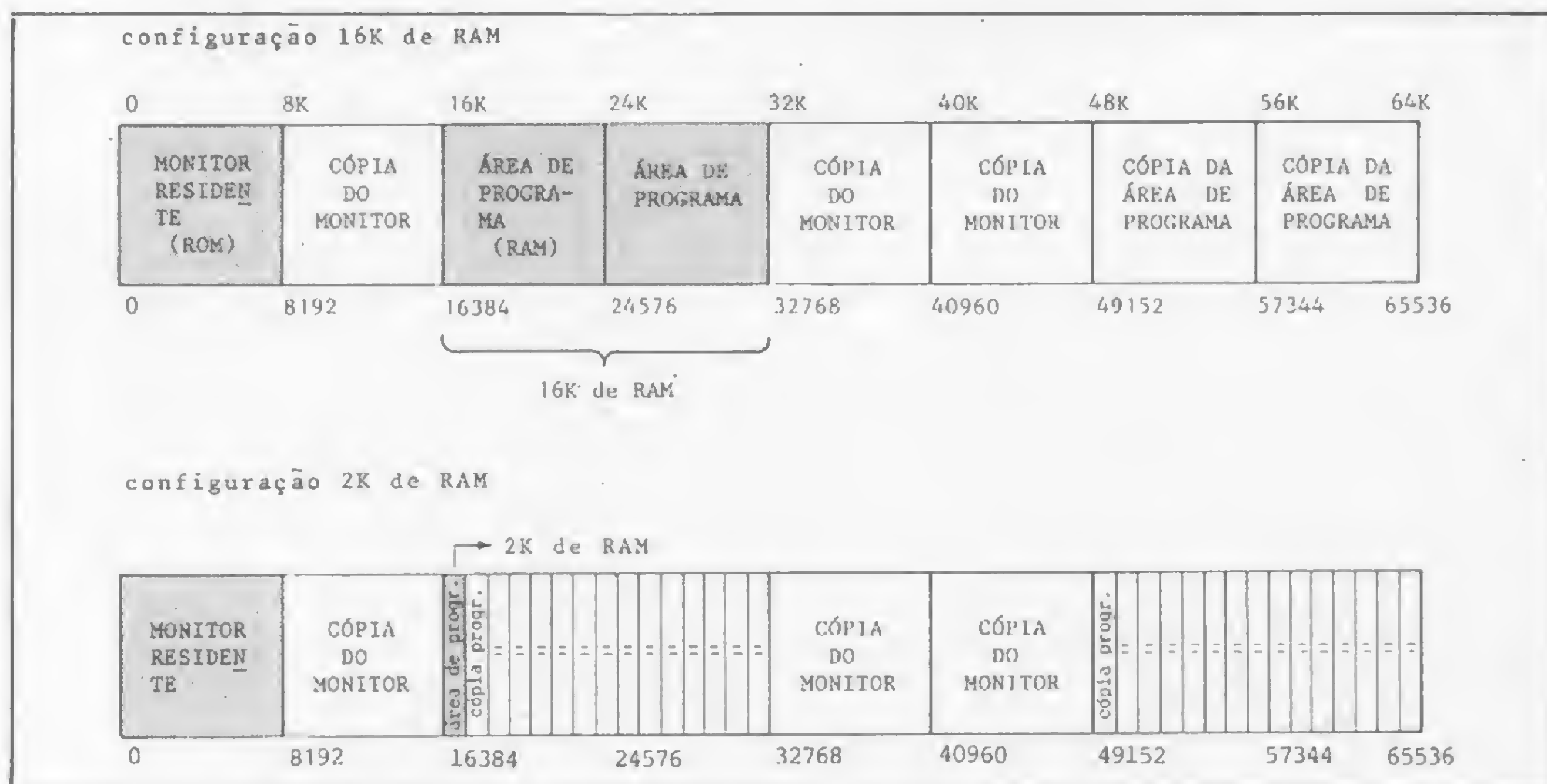
Figura 1 — Organização da memória
